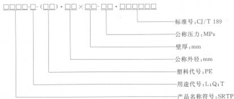
图 2 管材标记图
